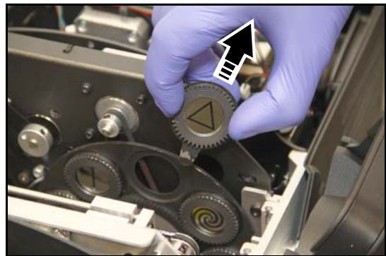
Bild 18: Entfernen eines Gobohalters aus Goborad 3
