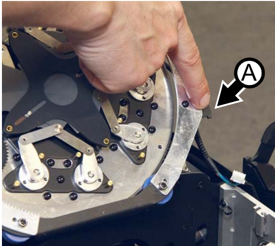
Bild 26: Führungsnut des Blendenschiebermoduls
