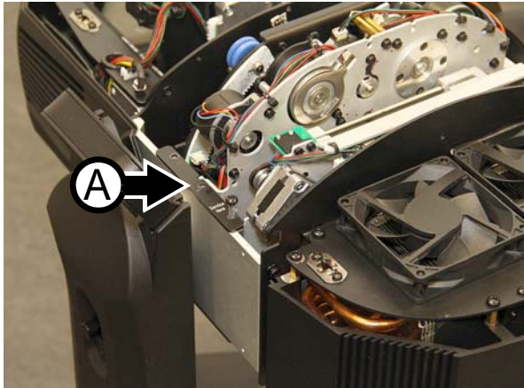
Bild 28: Installation der Halteleisten und des Lüfters
