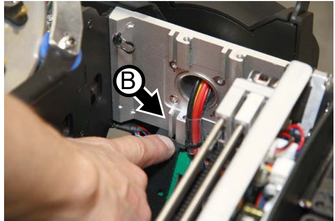
Bild 26: Führungsnut des Blendenschiebermoduls
