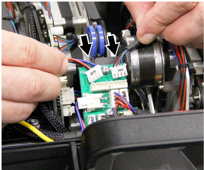
Bild 29: Anschließen des Effektmoduls
