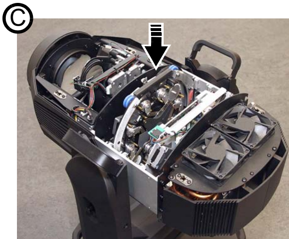
Bild 27: Installation des Blendenschieber- und Haupt-Effektmoduls
