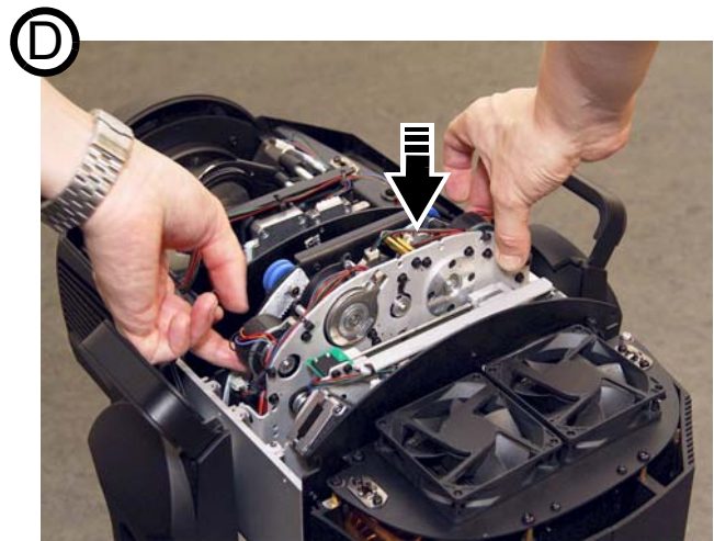
Bild 27: Installation des Blendenschieber- und Haupt-Effektmoduls
