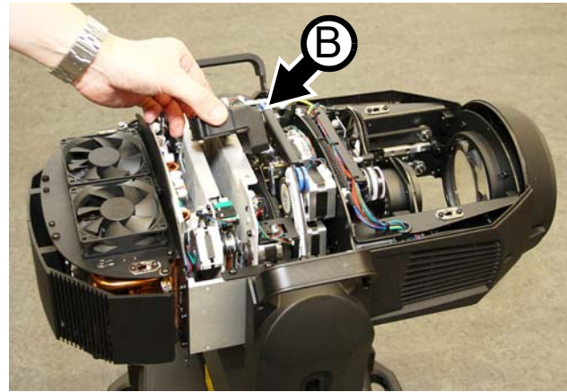
Bild 28: Installation der Halteleisten und des Lüfters
