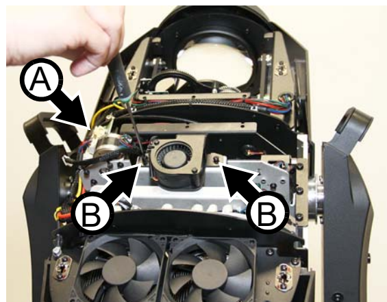
Bild 23: Entfernen des Lüfters des Effektmoduls
