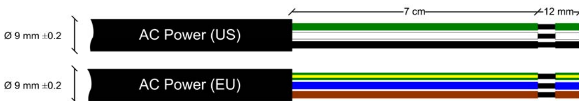
Câble d’alimentation
