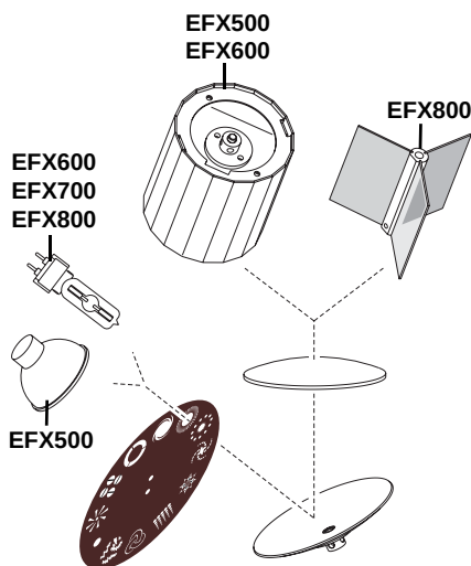
Composants optiques
