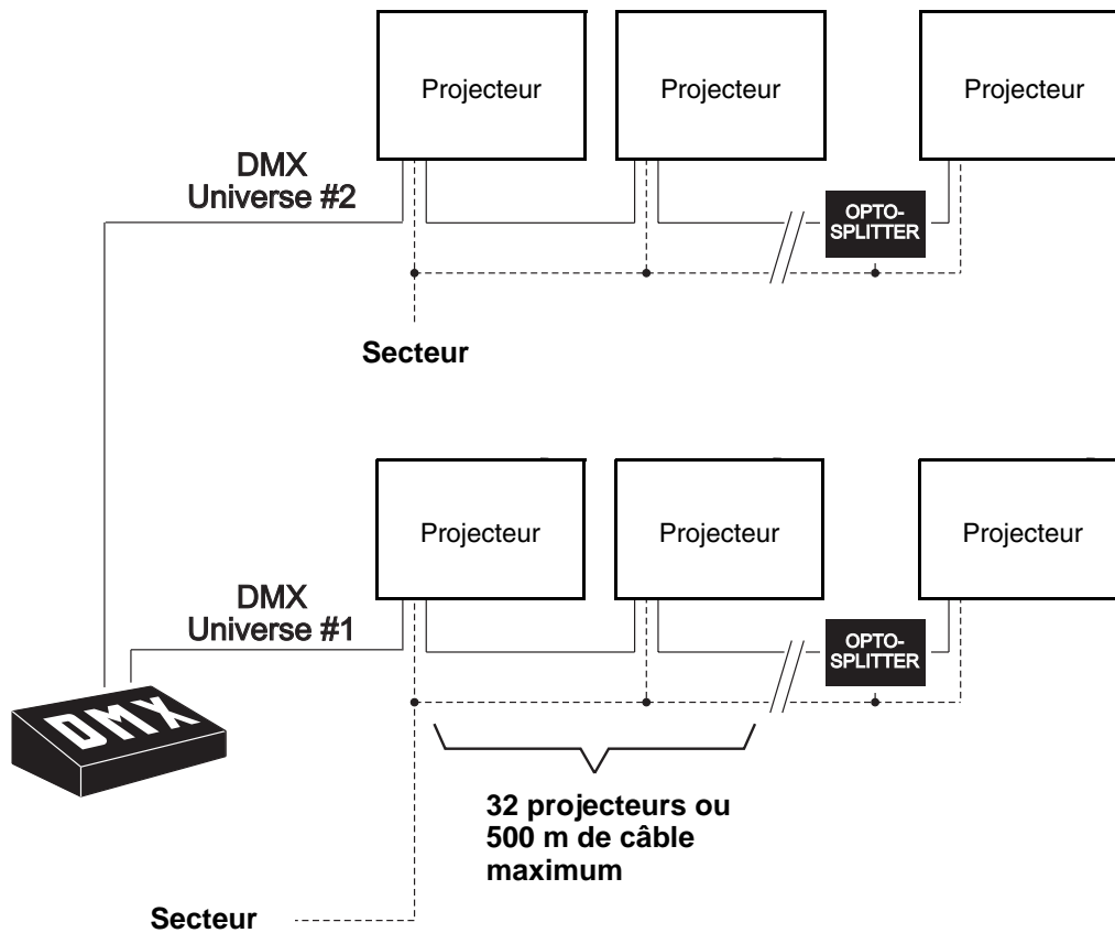
Figure 3: Synoptique de câblage
