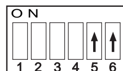
Réglage des DIP Switch pour le mode Boot Sector
