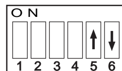
Réglage normal des DIP Switches
