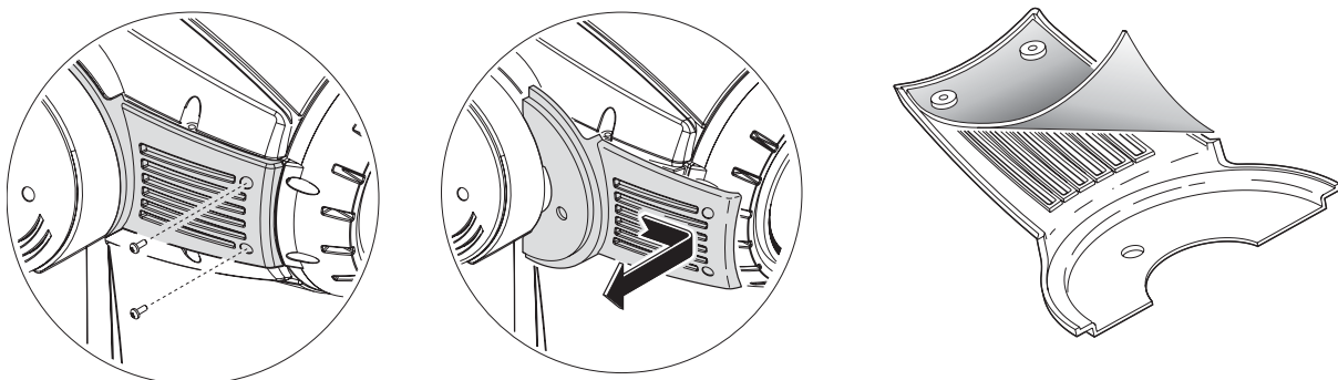
Bild 14: Entfernen der Luftfilter
