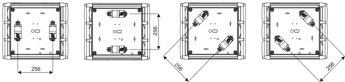
Bild 8: Montagepositionen der Camlock-Adapter
