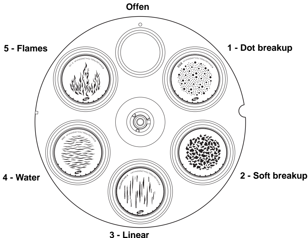
Bild 11: Standardbestückung der rotierenden Gobos, vom Leuchtmittel aus gesehen.
