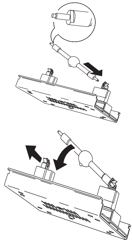
Bild 6: Einbau des Leuchtmittels
