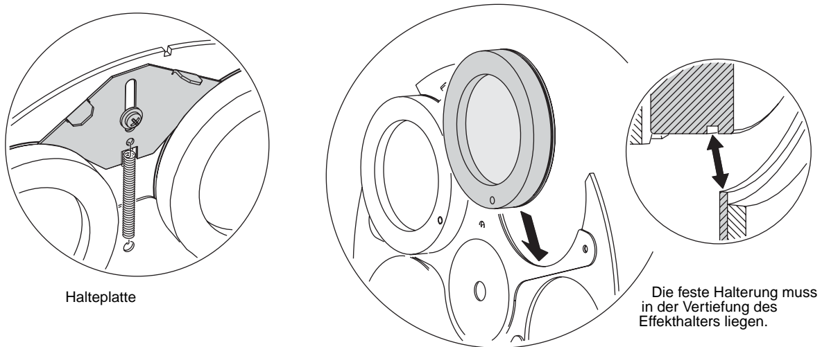
Bild 13: Austausch eines Effekts
