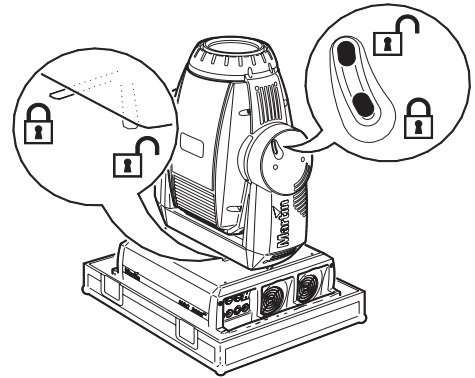
Bild 1: Transportsicherungen
