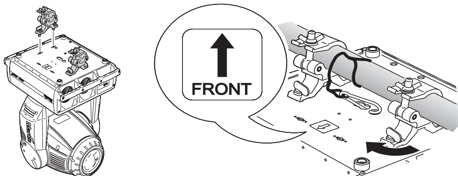
Bild 9: Montage der Befestigungsklemmen
