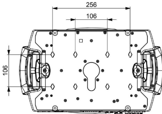
底座直角回转插座的尺寸
