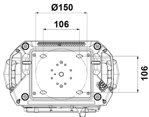
Bild 4: Befestigung der Omega-Adapter
