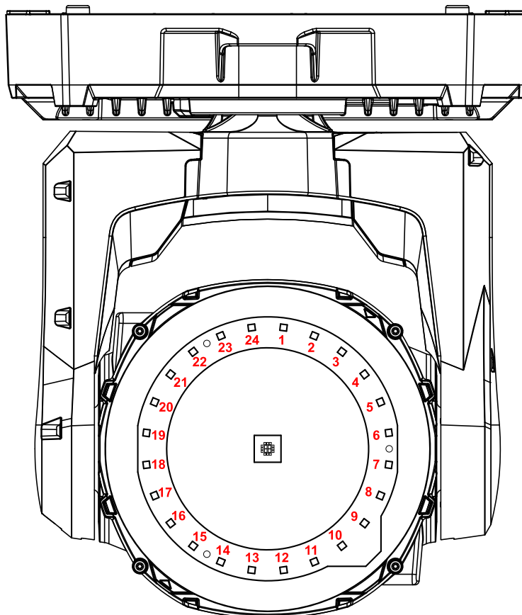
Distribución píxeles Backlight en MAC One
