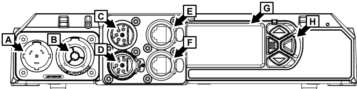
Panel de conexiones, panel de control
