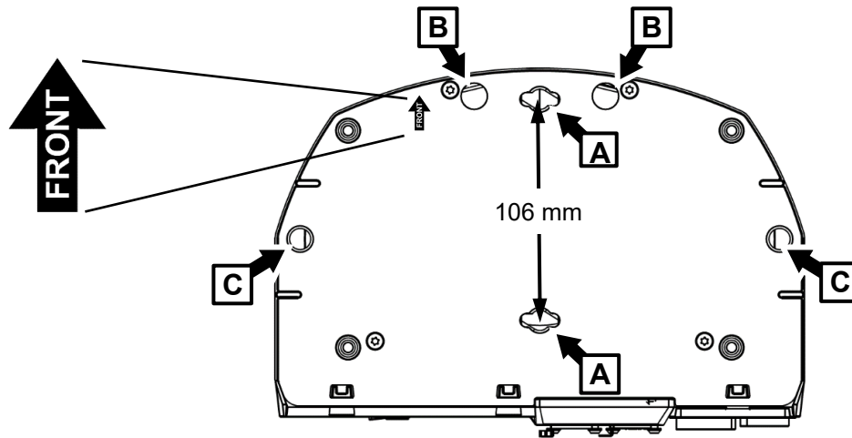
Base del dispositivo MAC One
