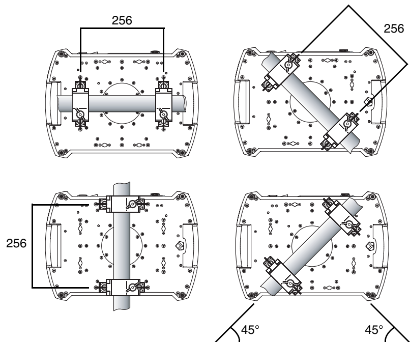
Bild 2: Mögliche Klemmenpositionen
