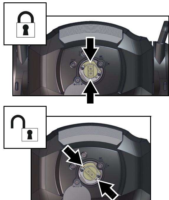
Bild 9: Leuchtmittel ver- / entriegeln
