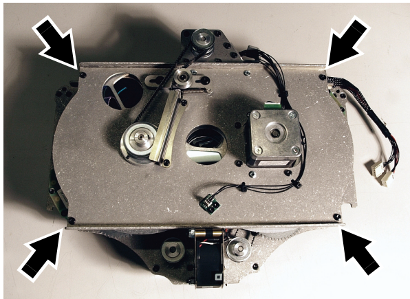
Bild 26: Öffnen des Projektionsmoduls
