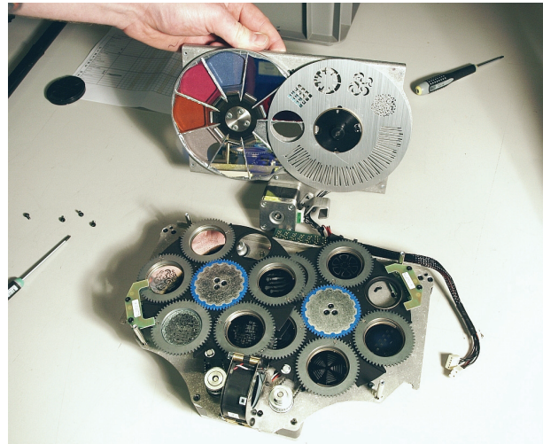
Bild 26: Öffnen des Projektionsmoduls
