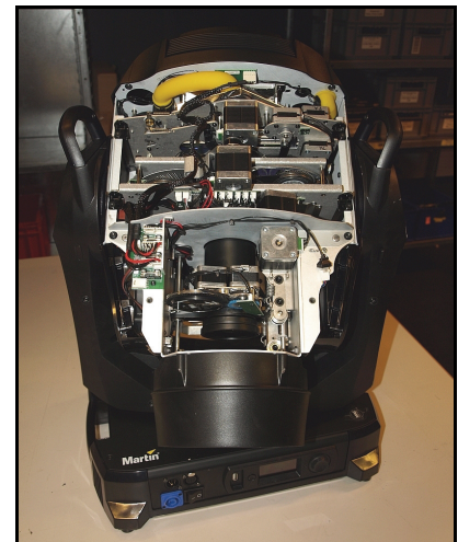
Bild 13: Günstige Wartungsposition des Kopfes
