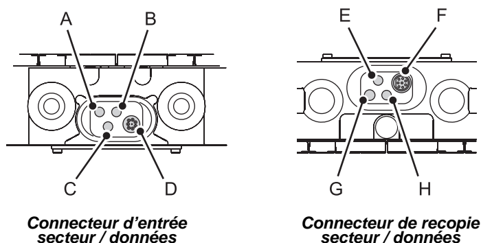
Figure 18: Connecteurs d'entrée et de recopie
