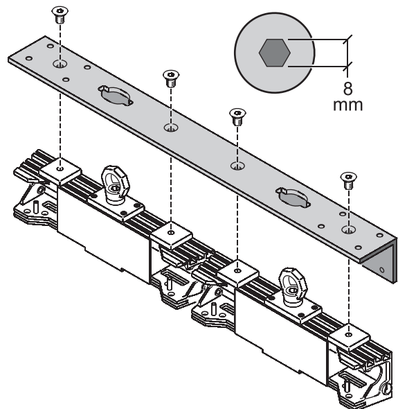
Figure 7: Coupleur de Blocs de Tête (Coupleur Double sur cette illustration)
