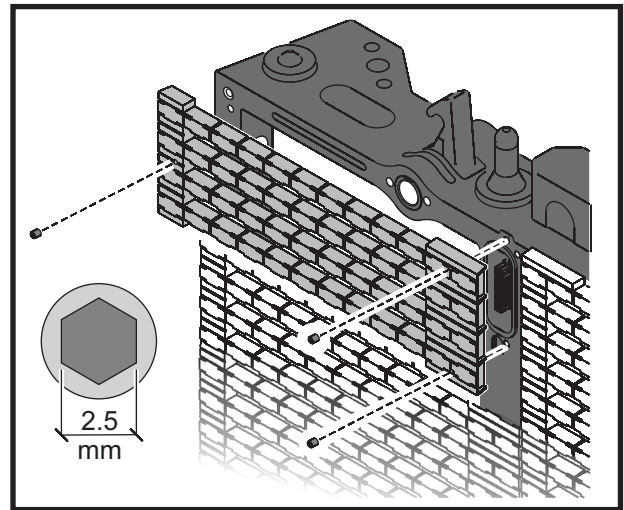
Figure 22: Remplacement d'un bloc de LEDs
