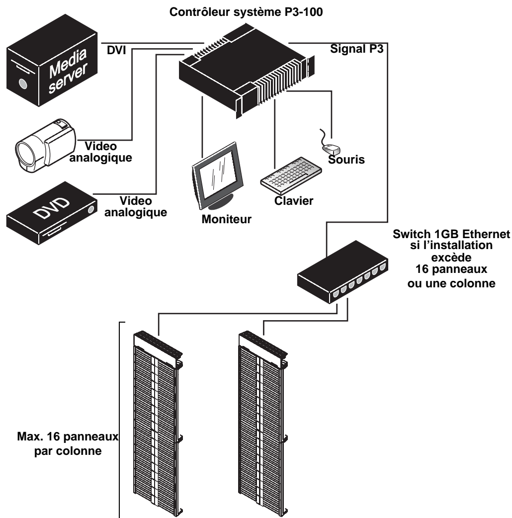
Figure 20: Diagramme schématique du réseau P3
