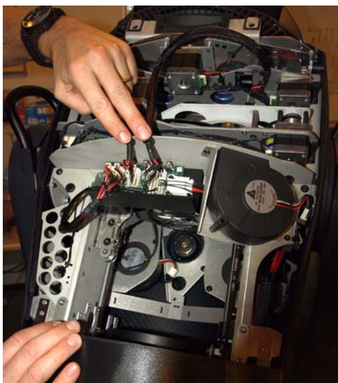
Figure 20: Connecteurs du module d'effets
