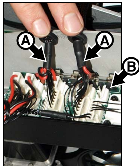
Figure 20: Connecteurs du module d'effets
