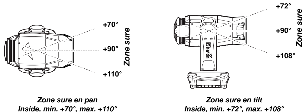
Figure 10: Réglage des limites de pan et tilt
