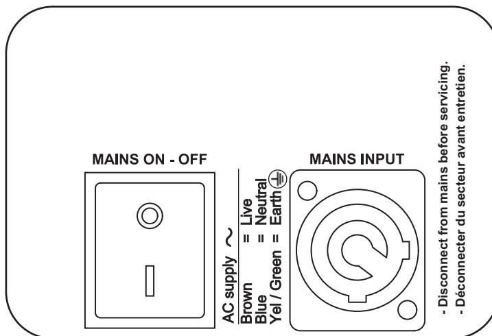
Figure 1: Connecteur secteur et interrupteur marche/arrêt
